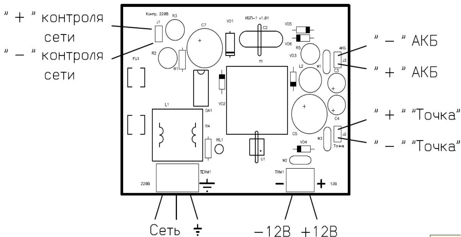
Рисунок 6.1 Схема подключения блока ИБП-1А v1.01
