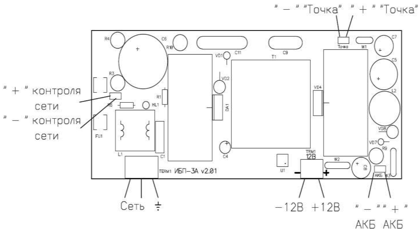
Рисунок 6.1 Схема подключения блока ИБП-5А v2.01
