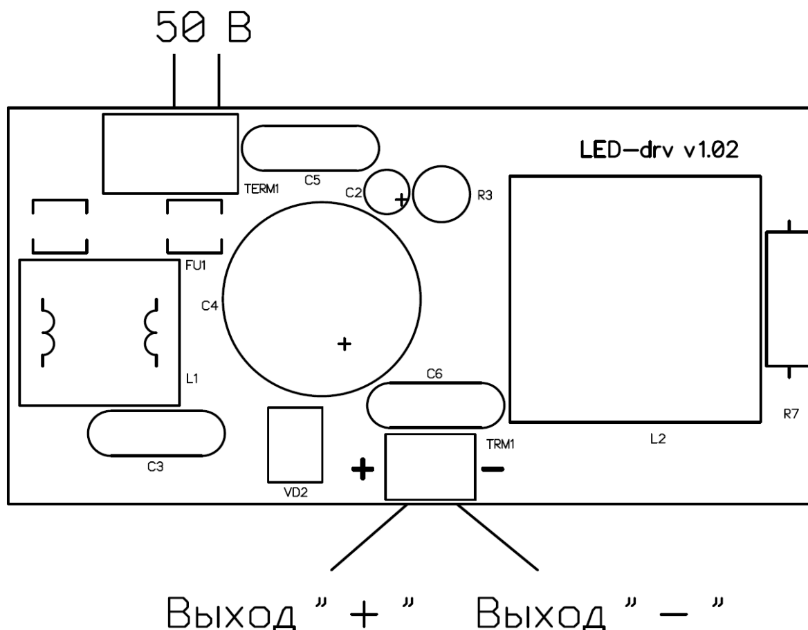
Рисунок 6.1 Схема подключения блока LED LED-3-50V
