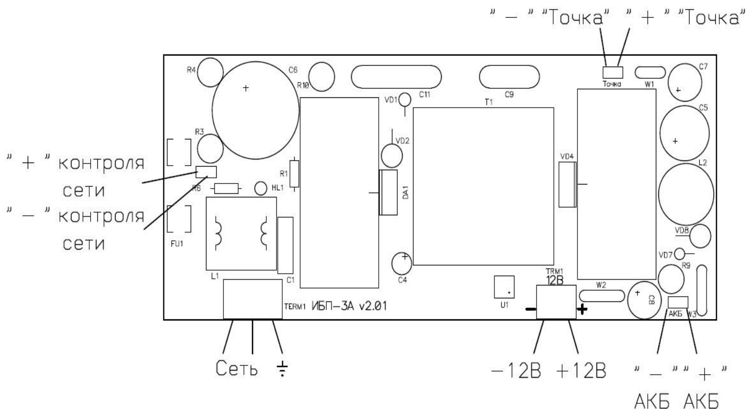
Рисунок 6.1 Схема подключения блока ИБП-3А v2.01
