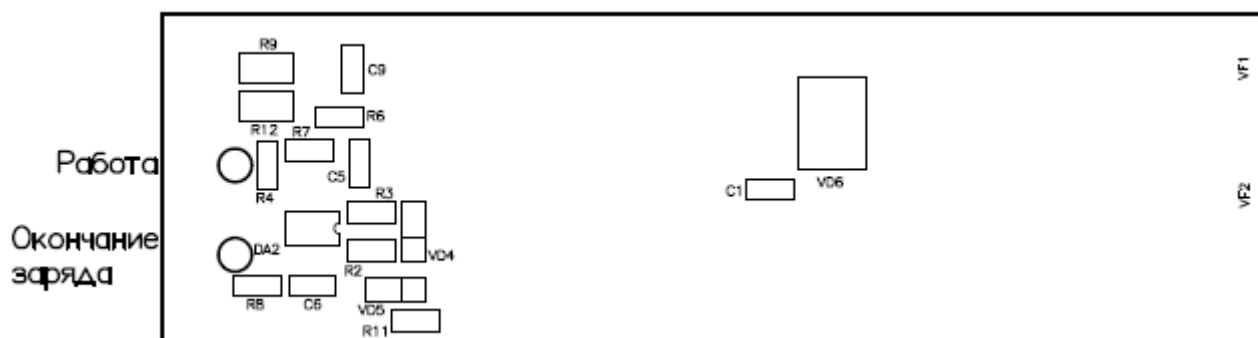
Рисунок 2. Расположение элементов индикации.
